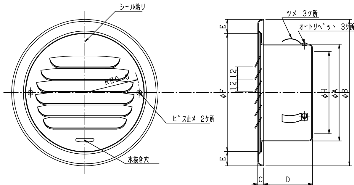
正面図
