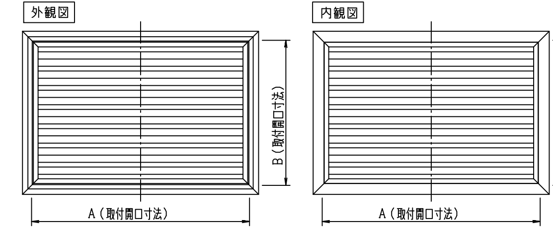
正面図
