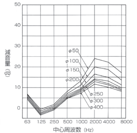
消音効果(1m)
