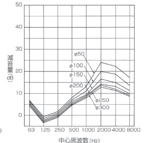
消音効果(1m)
