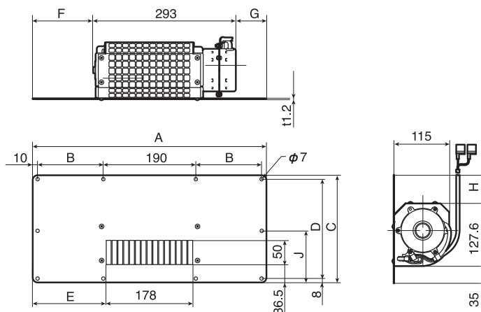
寸法表
