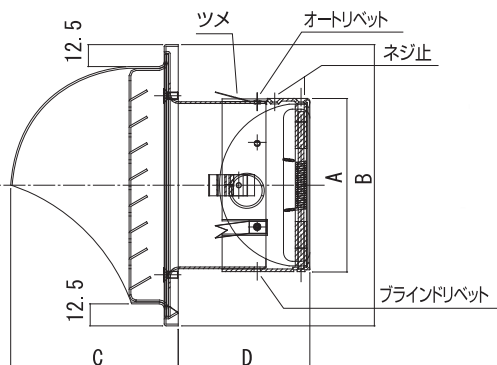
[縦断面図]
