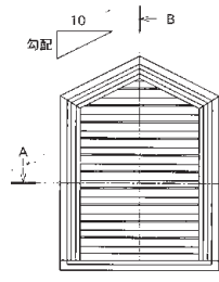
正面図
