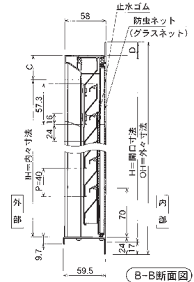
B-B断面図
