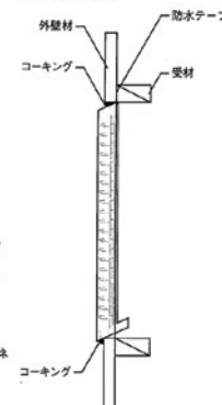
■ 取付参考図
