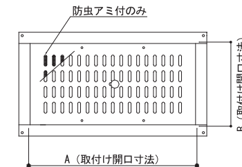
【外観図】
