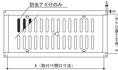
【外観図】
