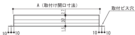
【外観図】
