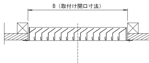
【施工例】
