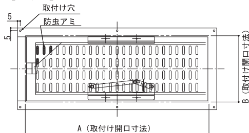
【外観図】
