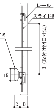
【縦断面図】
