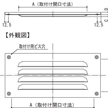
【横断面図】
