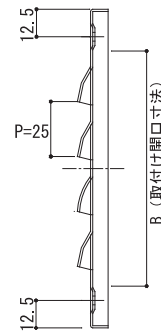
【縦断面図】
