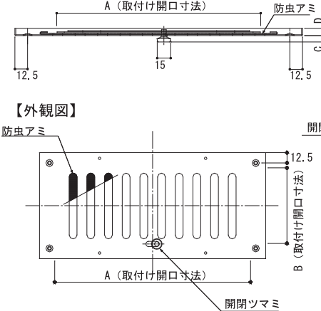
【横断面図】
