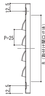
【縦断面図】
