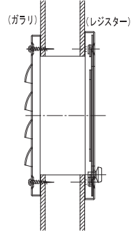
【施工例】
