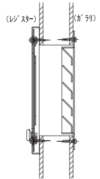
【施工例】
