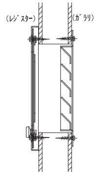
【施工例】
