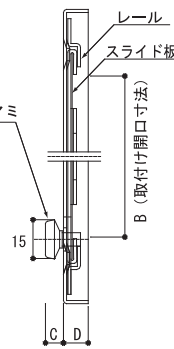
【縦断面図】
