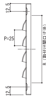
【縦断面図】
