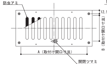
【外観図】
