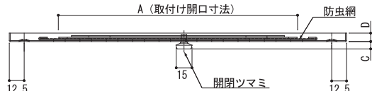
【外観図】
