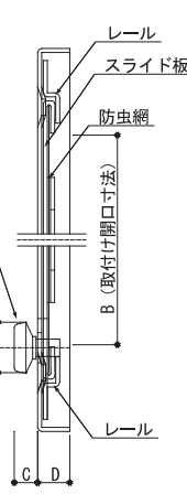
【縦断面図】
