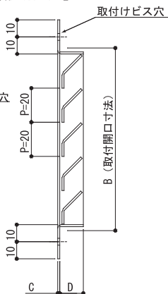
図面は3012サイズです
