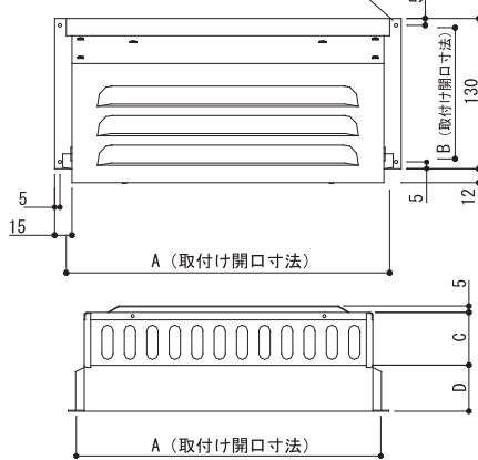
【外観図】
