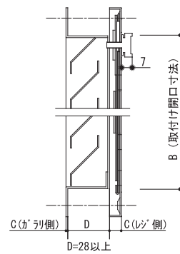
【縦断面図】
