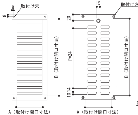
【外観図】
