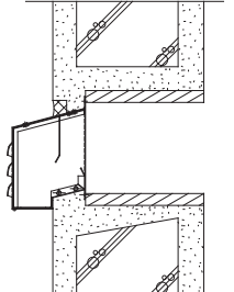
【施工例】
