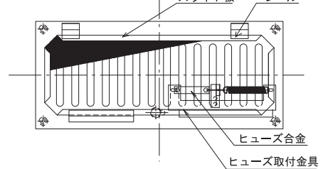
【レジスタ裏面図】
