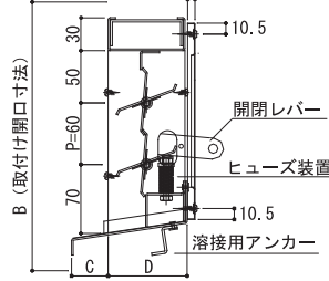
【縦断面図】
