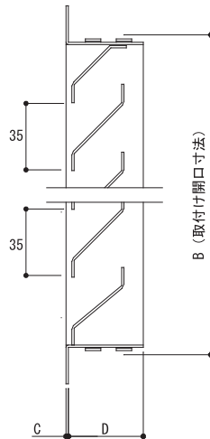
■ ZL-SUS型 寸法表
