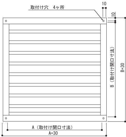
【外観図】
