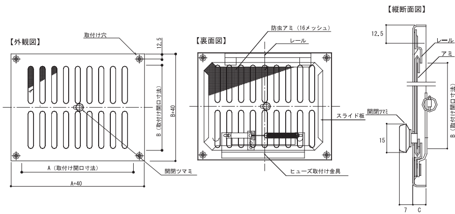
■104型FDスチール 寸法表
