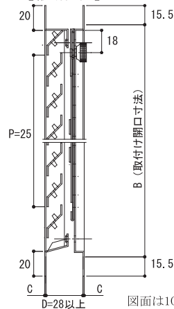
【縦断面図】
