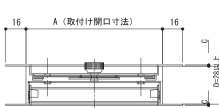
【横断面図】
