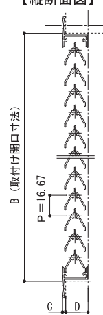
【縦断面図】
