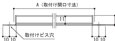
【外観図】
