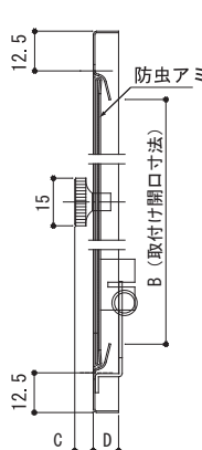
【縦断面図】
