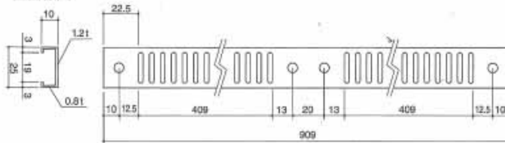
■ 仕様図
