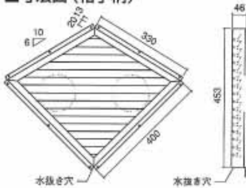
■寸法図(格子柄)
