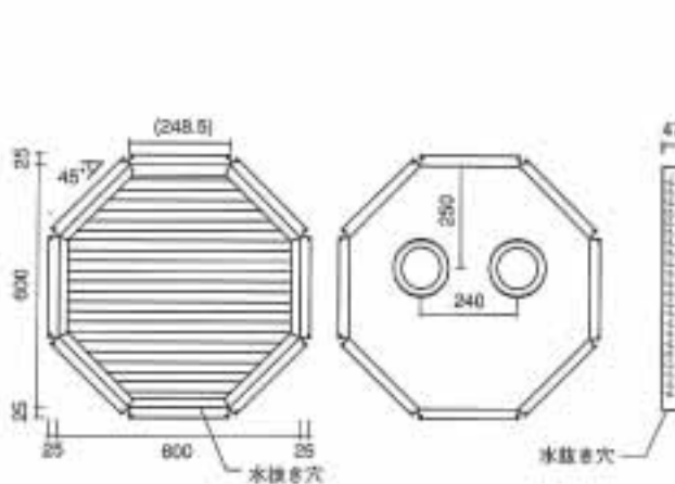
■寸法図
