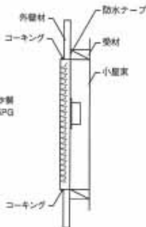
■取付参考図
