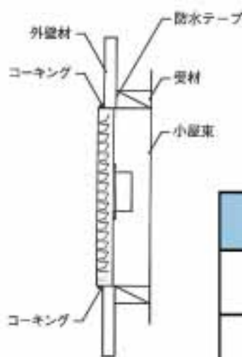
■取付参考図
