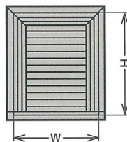
CSVO-A型 規格サイズ番号表(開口寸法)
