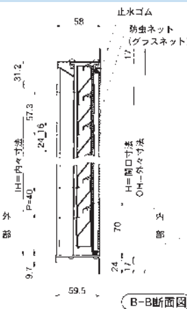
B-B断面図
