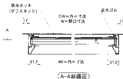
A-A断面図
