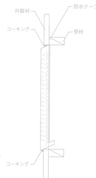
■ 取付参考図
