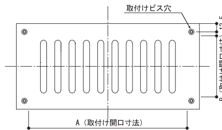
【外観図】
